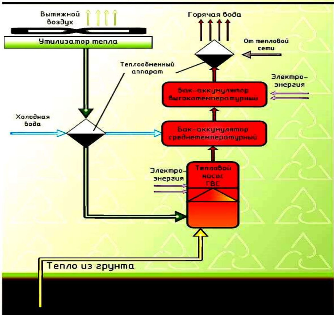
Рисунок 8 – Комбинированное использование теплоты вентиляционных выбросов и грунтового массива
