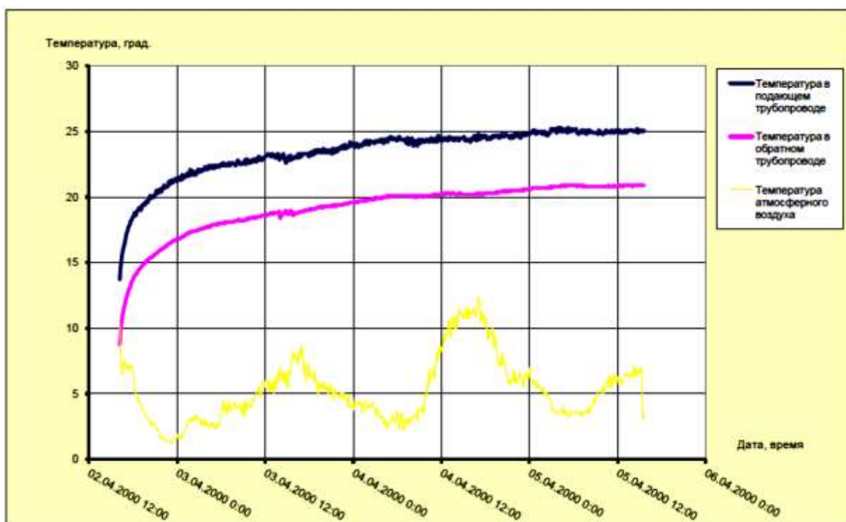
Рисунок А.2 – Графики температуры в подающем и в обратном трубопроводах, а также температуры атмосферного воздуха
