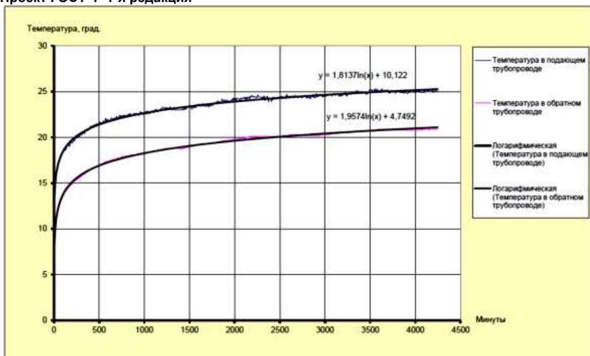
Рисунок А.3 – Логарифмическая аппроксимация трендовыми линиями графиков температуры в подающем и в обратном трубопроводах
