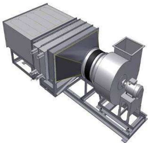
Рисунок 3 – Общий вид агрегата утилизации теплоты вентиляционных выбросов
