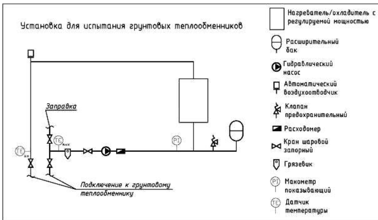
Рисунок А.1 – Пример схемы установки для проведения тепловых испытаний грунтовых теплообменников
