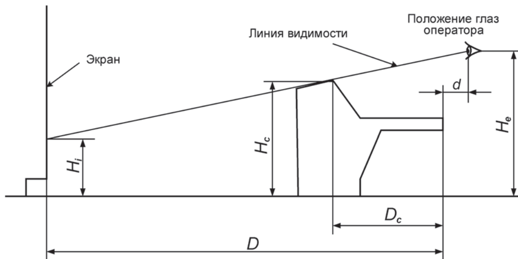
Рисунок П.6 – Элементы оборудования АРМ
